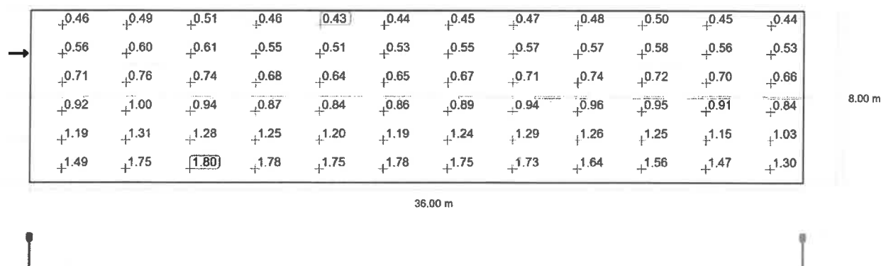
Observator 2: Valoarea de întreținere, densitatea luminii cu carosabil uscat [ \text{cd/m}^2 ] (Linii Isolux)
