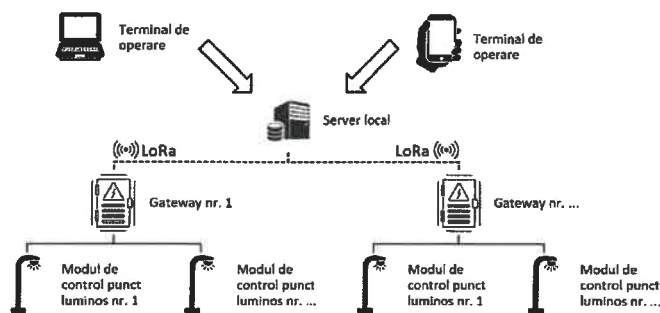
(Schema principiu de funcționare)
